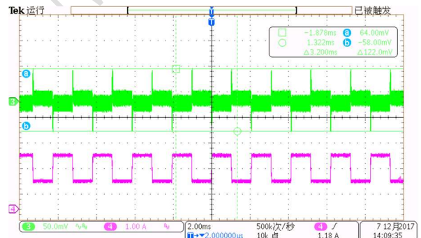
Load transient(1A-2A-1A)
