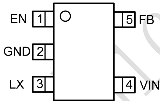
SOT23-5
