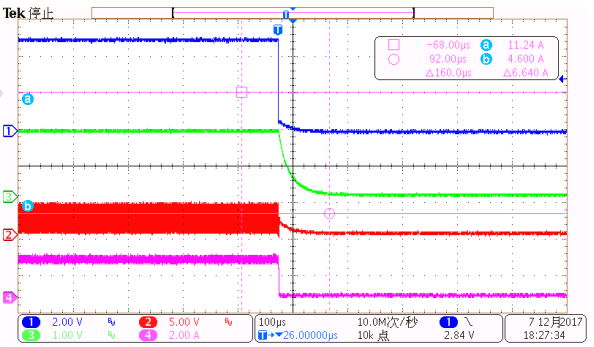
EN off, Iout= 2A
