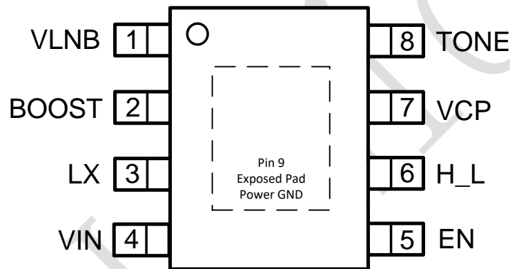
ESOP8
