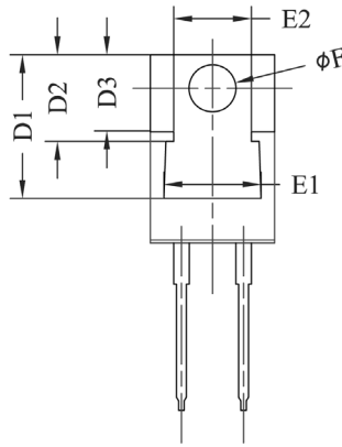
View A-A
