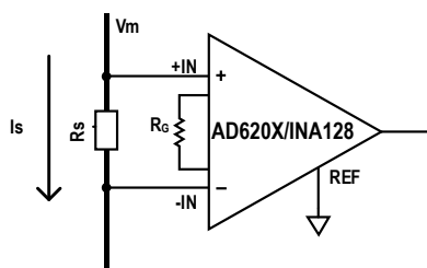
图 36. AD620X, INA128X 用于精密电流检测
