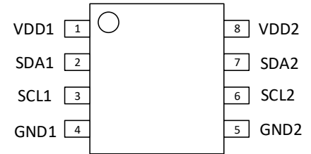
图 3. ISO1540/1640 引脚配置
