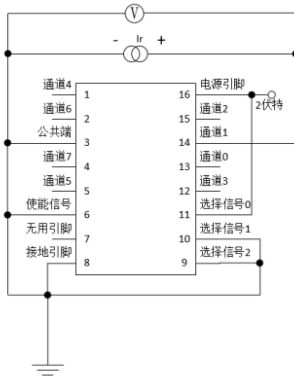
图6.1a 通道1正向开关电阻测试设置
