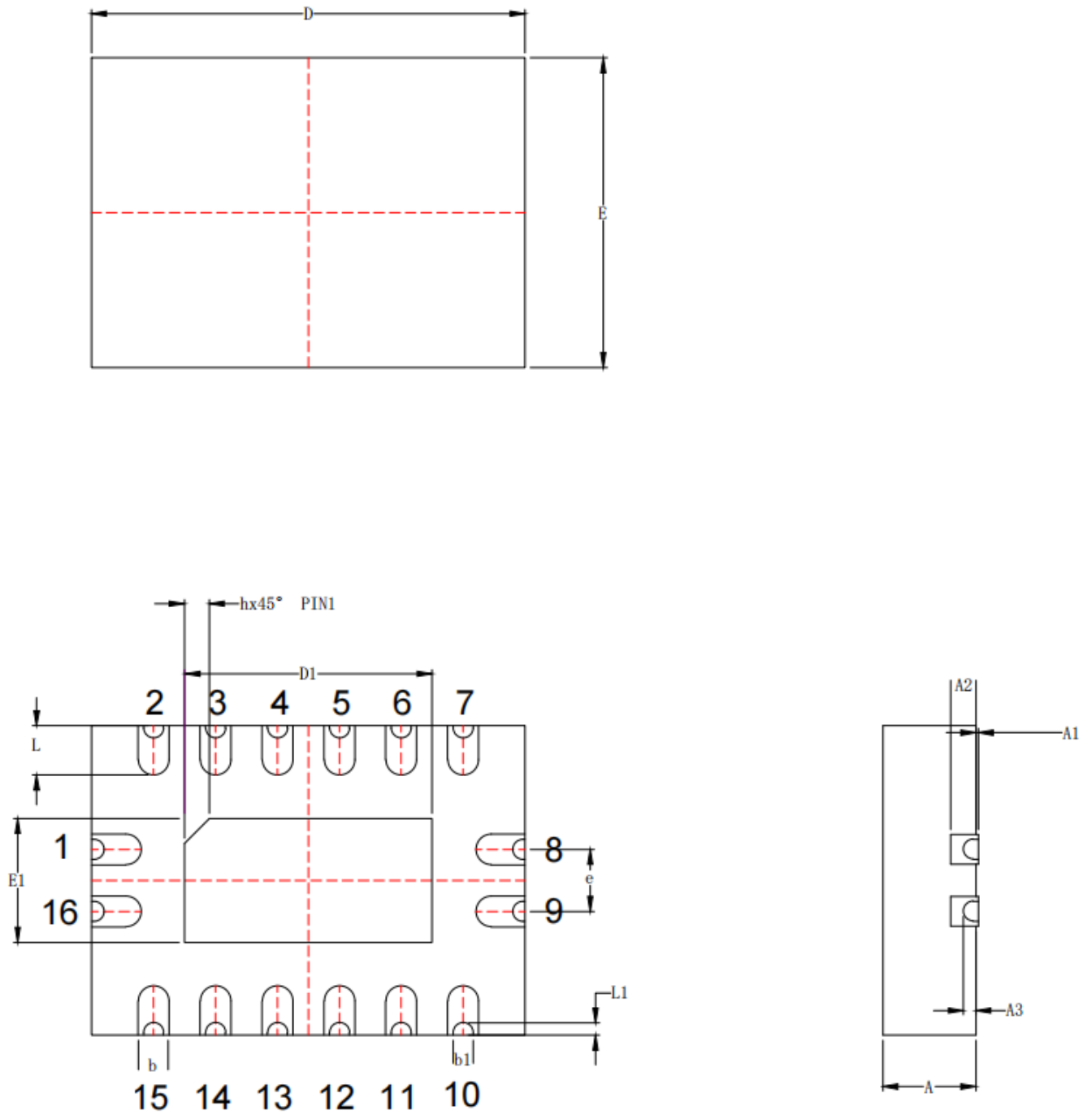
图9.2 QFN16 封装外形尺寸
