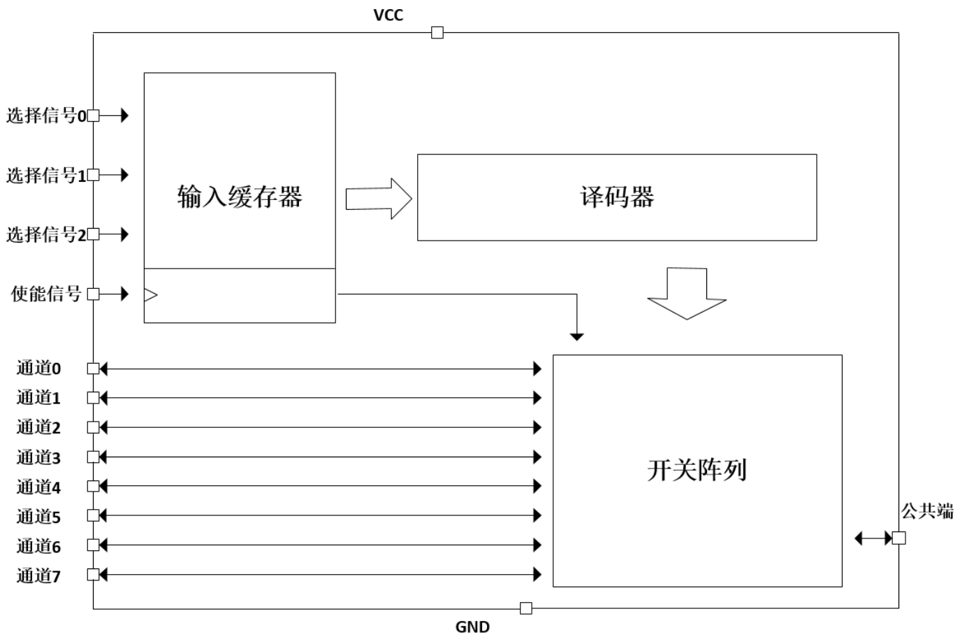
图7 功能模块框图
