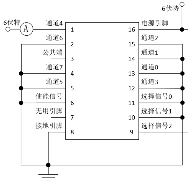
图6.2.3a 开启通道4到VCC的漏电流测试设置
