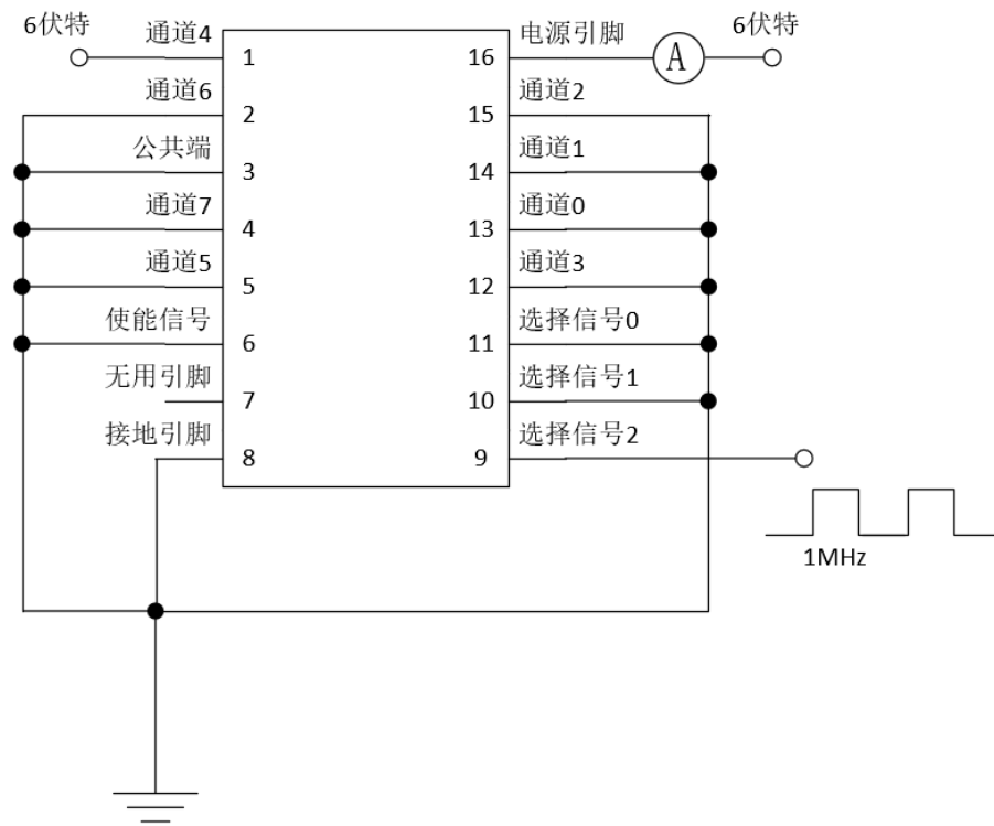
图6.5.2 动态工作电流测试设置
