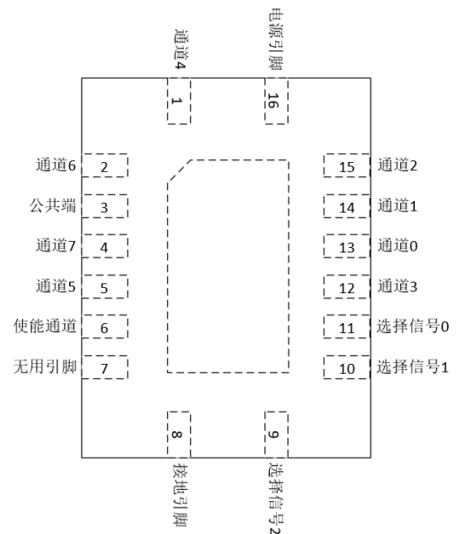
图4.2 QFN16引脚示意图
