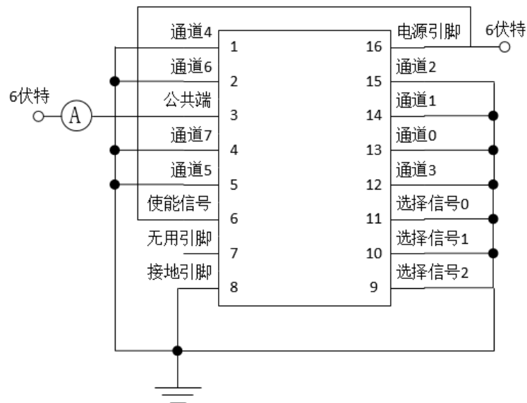
图6.2.2a 公共端到VCC的漏电流测试设置
