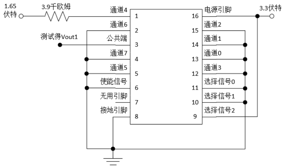
图6.3a 开启通道4和关断通道6最大偏移电压测试设置
