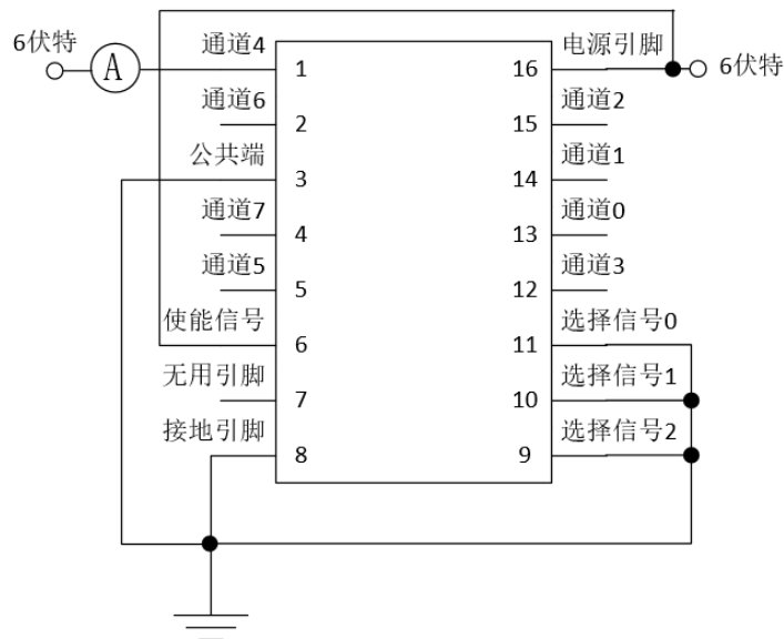
图6.2.1b 关断通道4到VCC的漏电流测试设置
