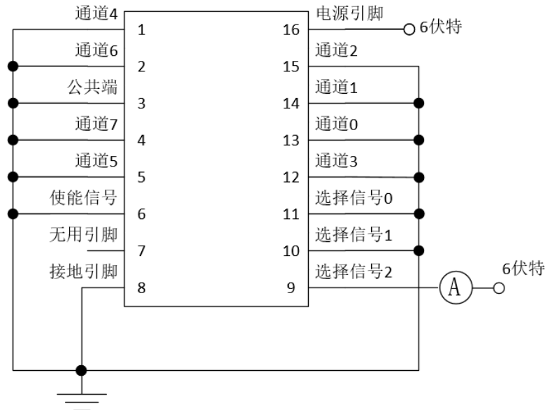
图6.2.4 选择信号2到VCC输入漏电流测试设置
