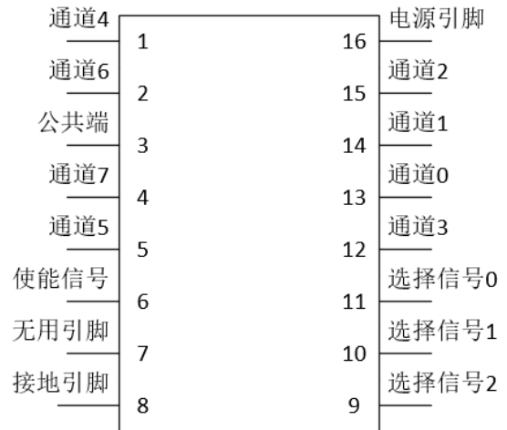
图4.1 TSSOP16引脚示意图
