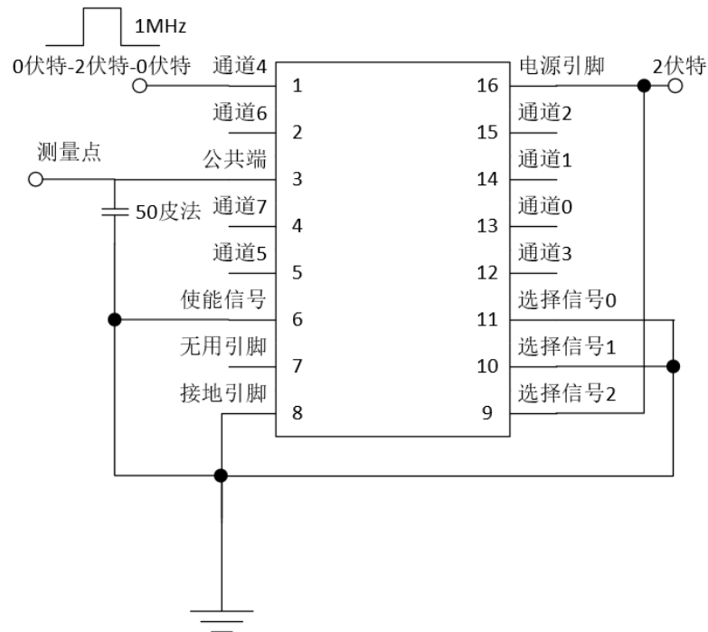
图6.4.2b 从开启通道到公共端传输延迟时间测试设置
