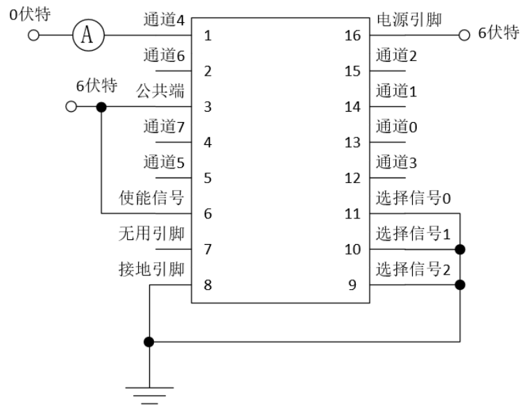
图6.2.1a 关断通道4到GND的漏电流测试设置
