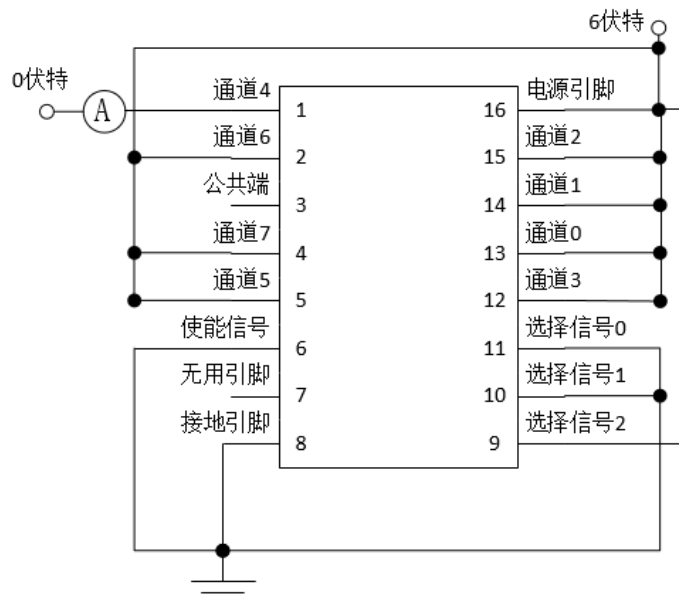
图6.2.3b 开启通道4到GND的漏电流测试设置
