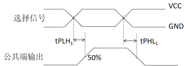
图6.4.1a 从选择信号到公共端传输延迟时间参数
