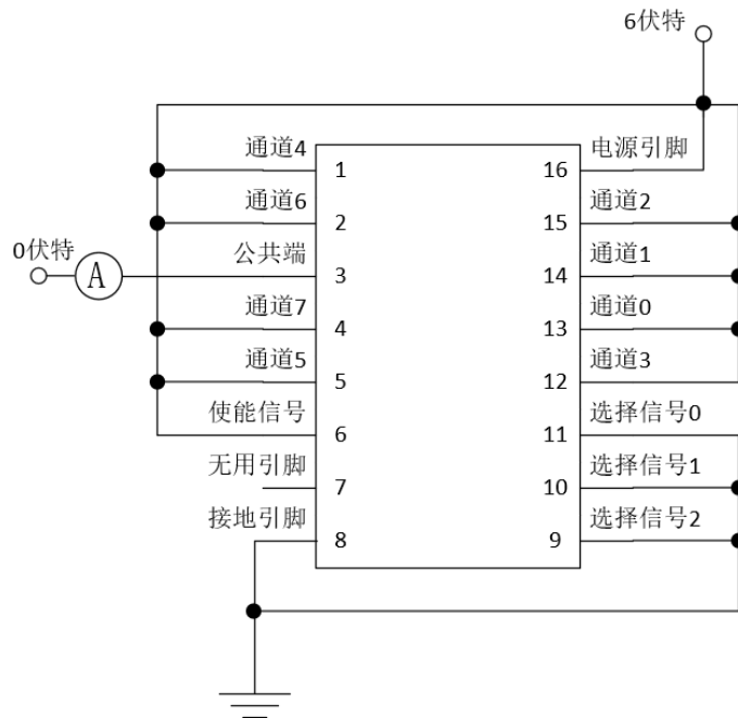
图6.2.2b 公共端到GND的漏电流测试设置
