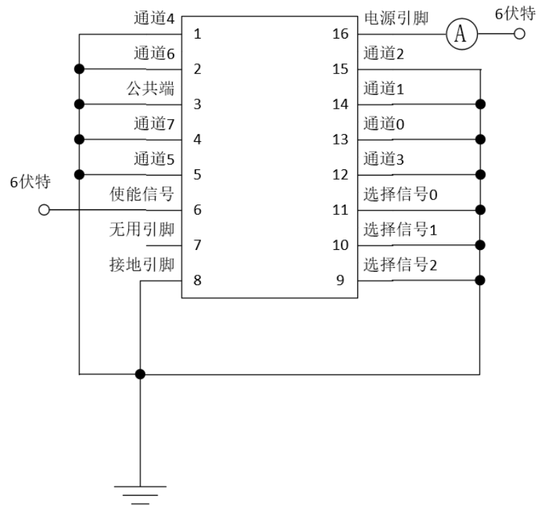
图6.5.1 静态工作电流测试设置
