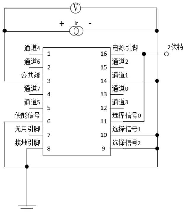
图6.1b 通道1反向开关电阻测试设置
