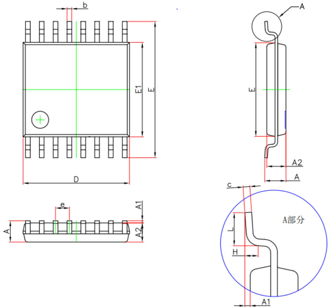
图9.1 TSSOP16 封装外形尺寸
