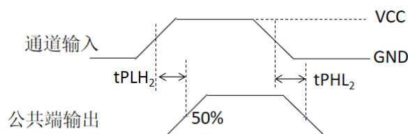
图6.4.2a从开启通道到公共端传输延迟时间参数
