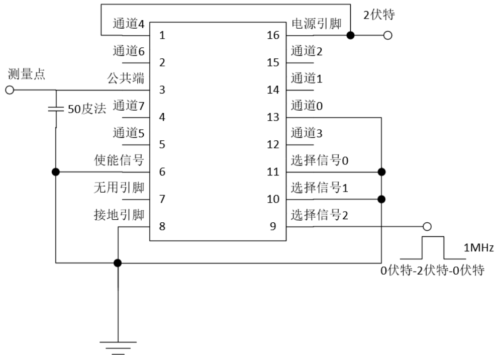
图6.4.1b 从选择信号到公共端传输延迟时间测试设置
