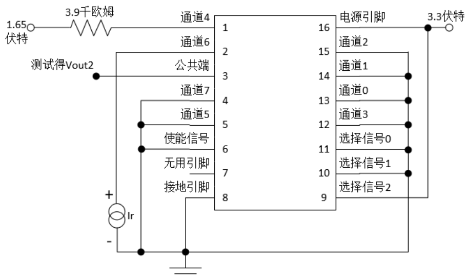
图6.3b 开启通道4和关断通道6最大偏移电压测试设置
