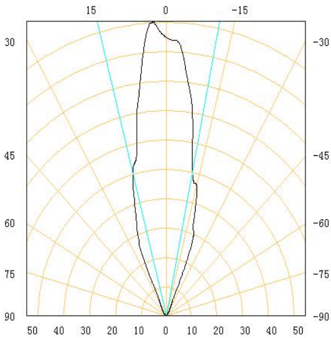
发射角度(Red)
