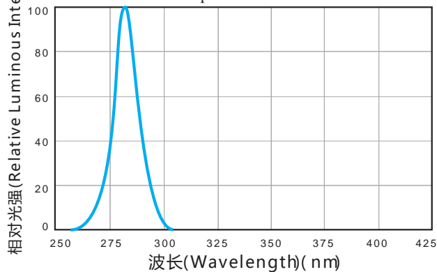
光谱分布特性曲线 Relative Spectral Distribution
