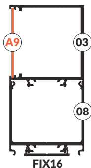
variant 32 - wall side FIX16-08-03-A9 wariant 32 - ścienny boczny FIX16-08-03-A9
