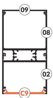
variant 27 - pendant 09-08-02-C9 wariant 27 - wiszący 09-08-02-C9
