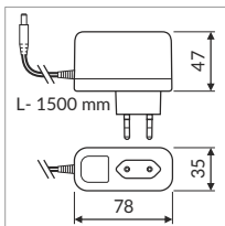
18 W 12 V / 100-240 V AC adapter / zasilacz wtyczkowy
