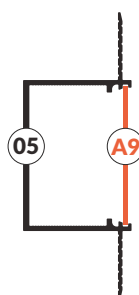
variant 05 - recessed 05-A9 spackle flange wariant 05 - wpustowy 05-A9 do szpachlowania
