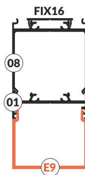
variant 15 - ceiling FIX16-08-01-E9 wariant 15 - sufitowy FIX16-08-01-E9
