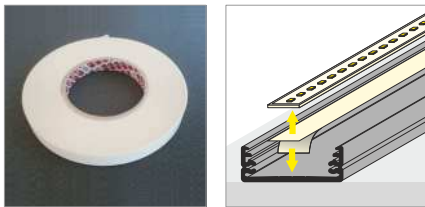
adhesive tape double-sided thermally conductive taśma dwustronna termoprzewodząca
