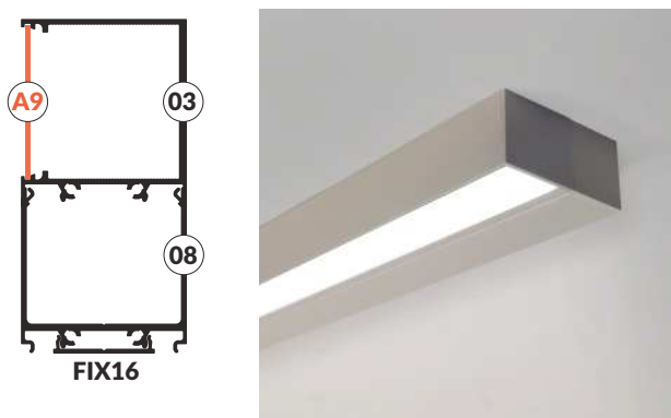
variant 32 - wall side FIX16-08-03-A9 wariant 32 - ścienny boczny FIX16-08-03-A9
