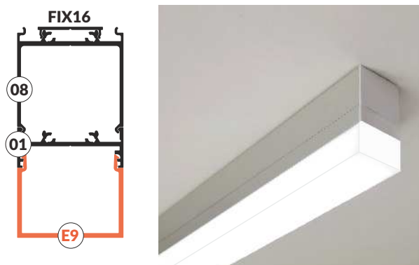
variant 15 - ceiling FIX16-08-01-E9 wariant 15 - sufitowy FIX16-08-01-E9
