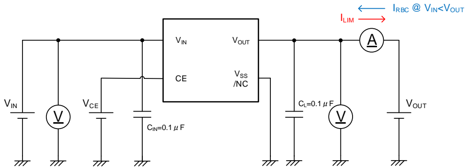
Test CIRCUITS③
