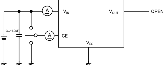
●Circuit②
