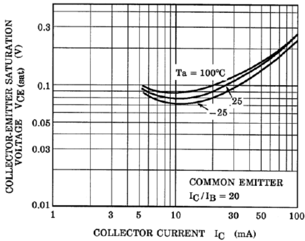
Fig. 10.19 RN1301 V_{CE(sat)}-I_C
