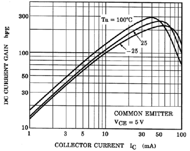
Fig. 10.14 RN1302 h_{FE}-I_C
