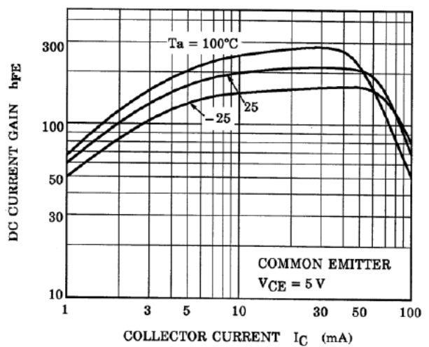
Fig. 10.18 RN1306 h_{FE}-I_C
