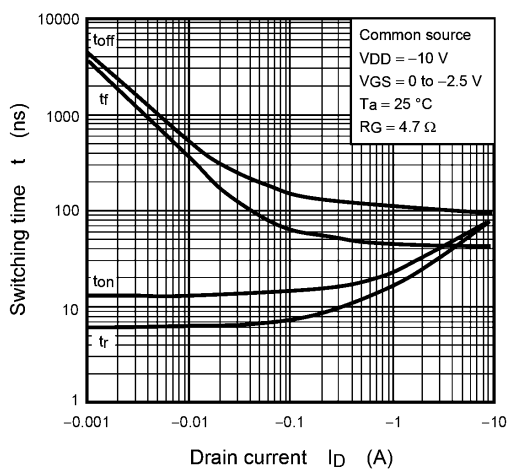
Fig. 8.11 t - I_D
