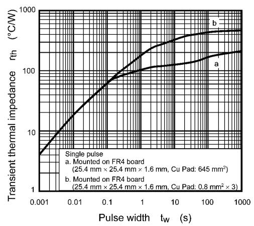
Fig. 7.12 r_{th} - t_w
