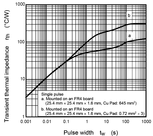
Fig. 8.12 r_{th} - t_w
