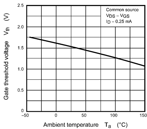
Fig. 8.6 V_{th} - T_a
