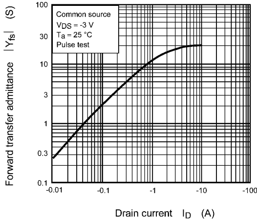
Fig. 7.7 |Y_{fs}| - I_D
