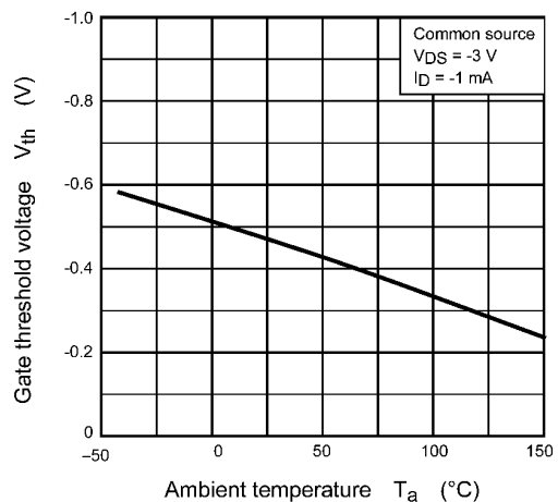
Fig. 7.6 V_{th} - T_a
