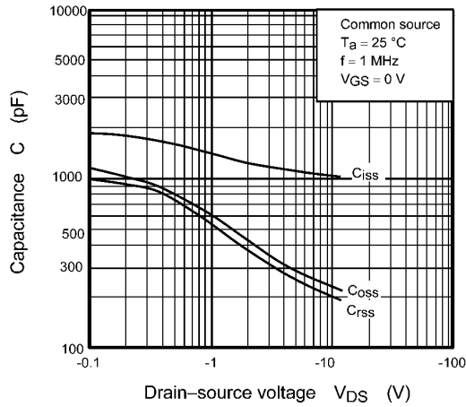
Fig. 7.9 C - V_{DS}
