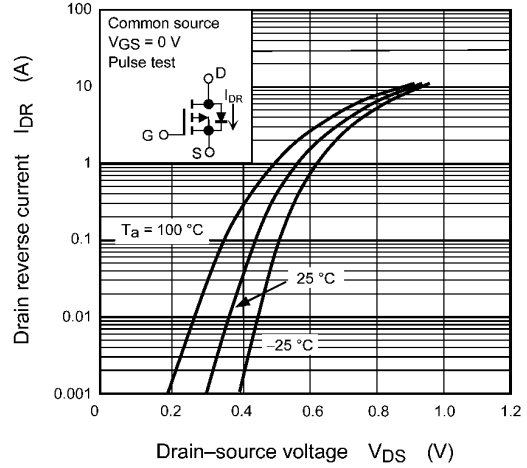
Fig. 7.8 I_{DR} - V_{DS}
