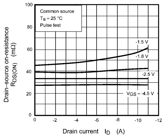
Fig. 7.4 R_{DS(ON)} - I_D
