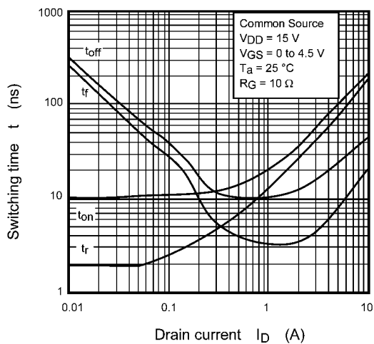
Fig. 8.11 t - I_D
