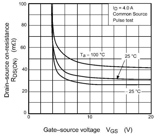
Fig. 8.4 R_{DS(ON)} - V_{GS}
