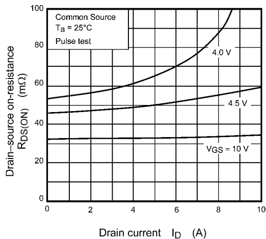
Fig. 8.5 R_{DS(ON)} - I_D
