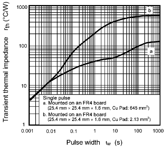
Fig. 8.13 r_{th} - t_w
