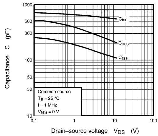
Fig. 7.10 C - V_{DS}
