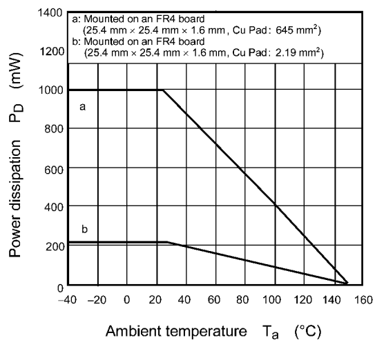
Fig. 7.14 P_D - T_a
