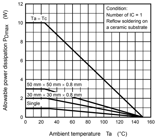
P_{Dmax} - T_a
