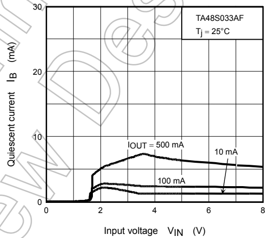
I_B - V_{IN}
