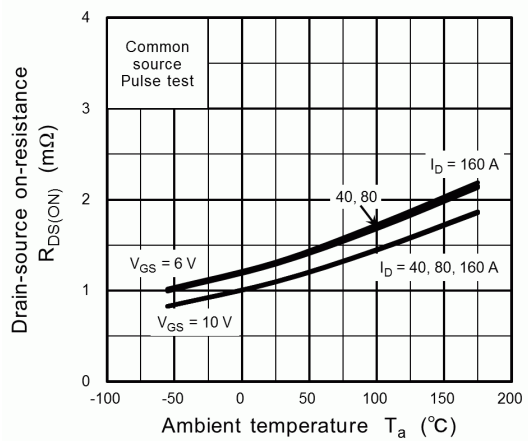
Fig. 9.6 R_{DS(ON)} - T_a
