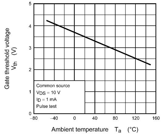
Fig. 8.10 V_{th} - T_a
