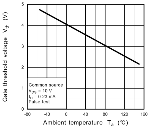
Fig. 8.11 V_{th} - T_a
