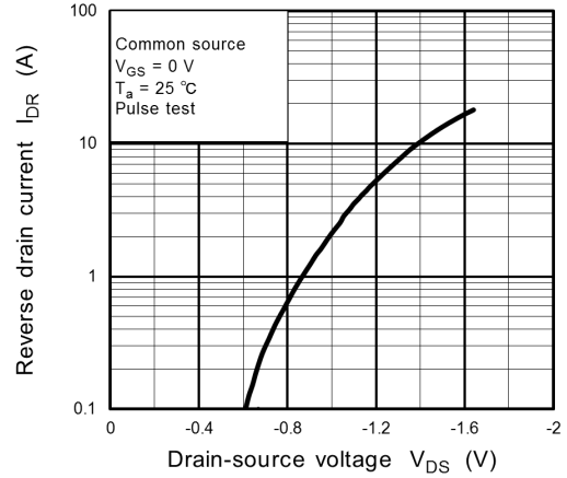
Fig. 8.8 I_{DR} - V_{DS}
