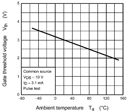
Fig. 8.11 V_{th} - T_a
