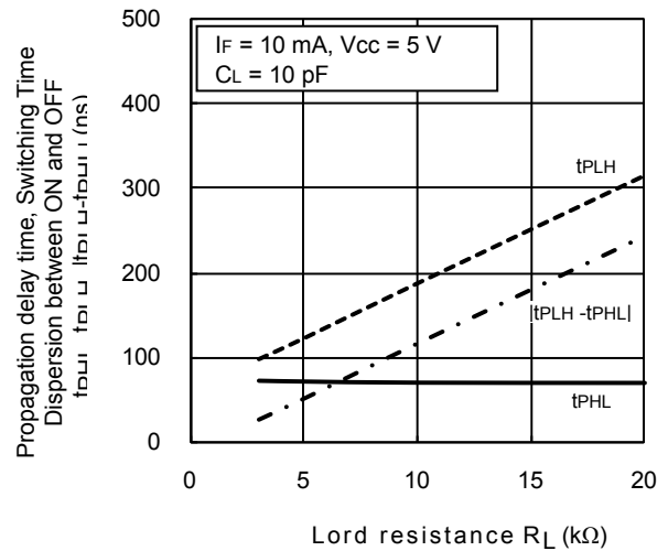
t_{PHL}/t_{PLH}/|t_{PLH}-t_{PHL}| - R_L
