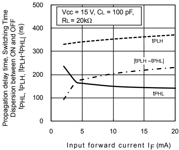
t_{PHL}/t_{PLH}/|t_{PLH}-t_{PHL}| - I_F
