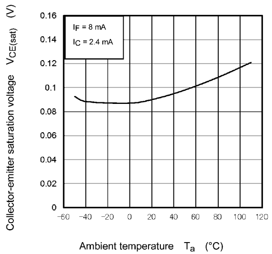
Fig. 11.12 V_{CE(\text{sat})} - T_a
