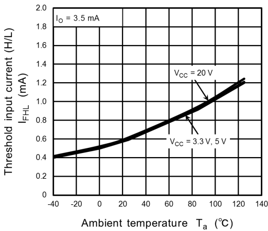
Fig. 12.2.11 I_{FHL} - T_a
