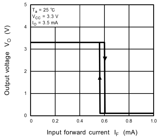
Fig. 12.2.12 V_O - I_F
