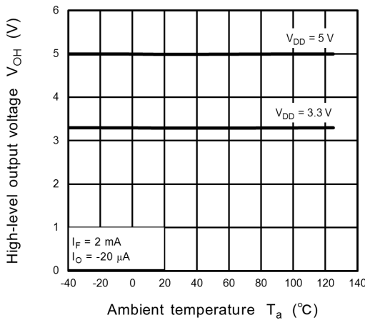
Fig. 13.2.5 V_{OH} - T_a
