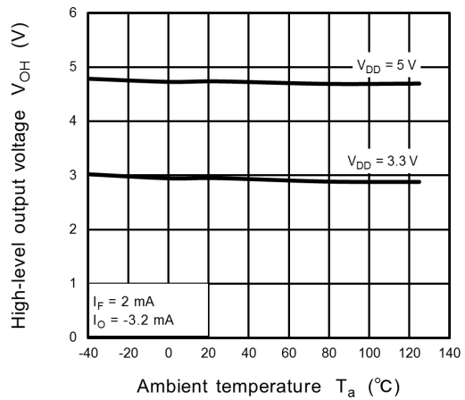
Fig. 13.2.6 V_{OH} - T_a
