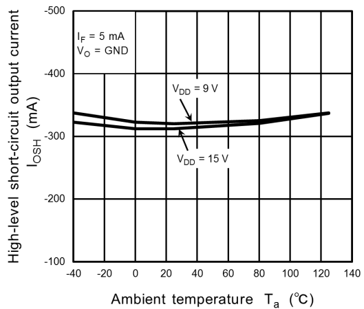
Fig. 12.2.10 I_{OH} - T_a
