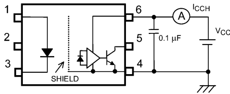
Fig. 13.1.3 I_{CCH} Test Circuit
