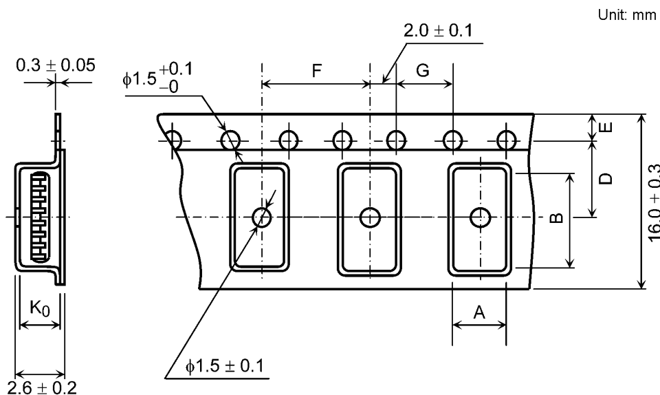
Fig. 15.3.5.1 Tape Dimensions
