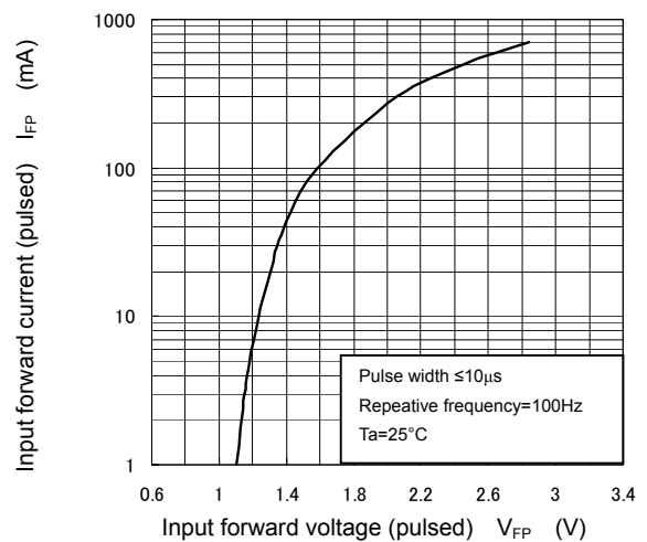
I_{FP} - V_{FP}
