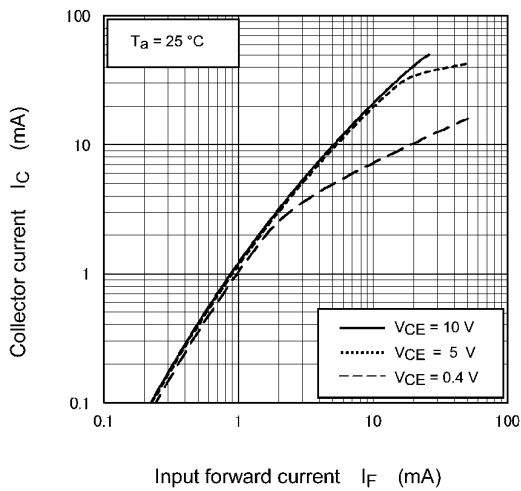
Fig. 11.11 I_C - I_F
