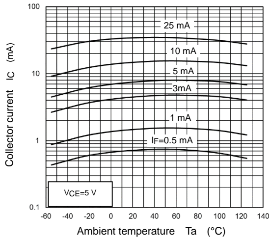
I_C - T_a
