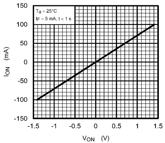
Fig. 12.4 I_{ON} - V_{ON}
