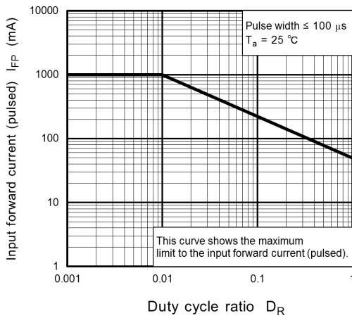
Fig. 11.3 I_{FP} - D_R
