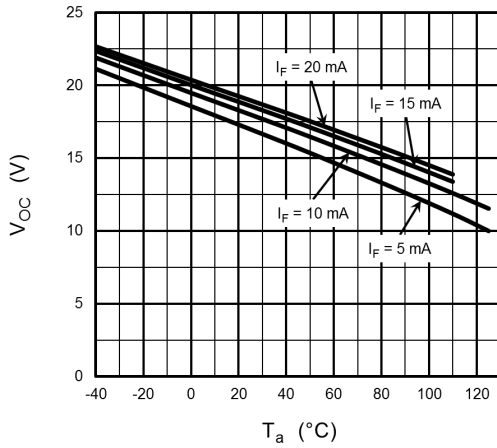
Fig. 12.7 V_{OC} - T_a
