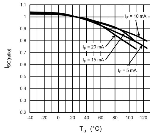
Fig. 12.10 I_{SC(ratio)} - T_a
