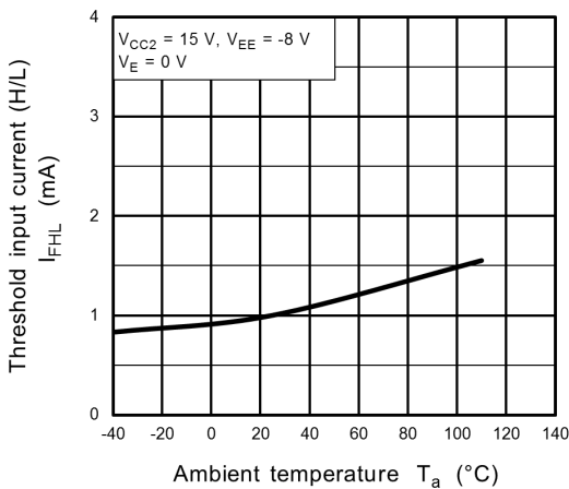
Fig. 13.3.29 I_{FHL} - T_a
