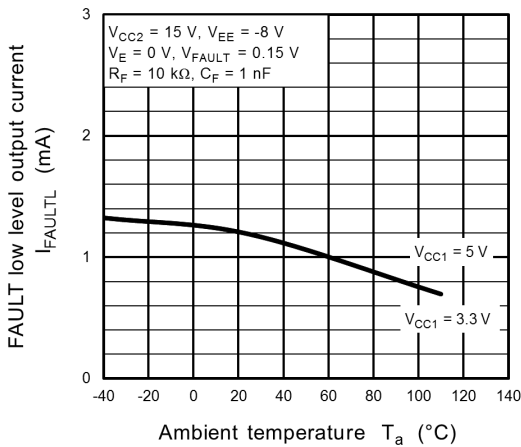
Fig. 13.3.27 I_{FAULTL} - T_a
