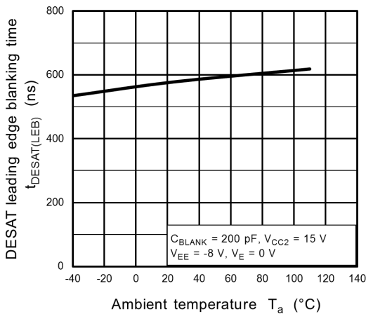
Fig. 13.3.35 t_{DESAT(LEB)} - T_a
