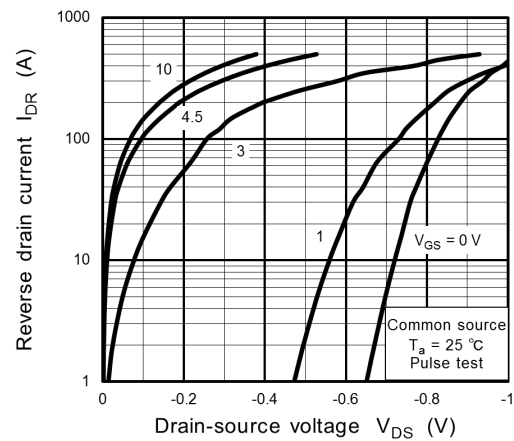
Fig. 8.6 I_{DR} - V_{DS}
