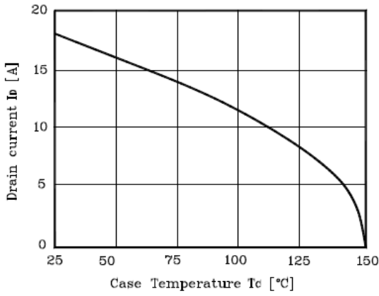
Fig. 9 I_D - T_C
