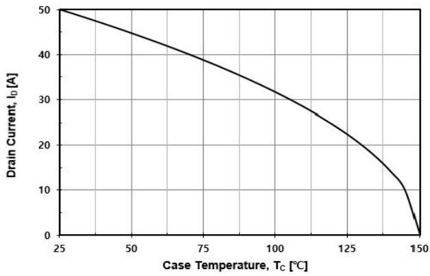
Fig. 9 I_D - T_C
