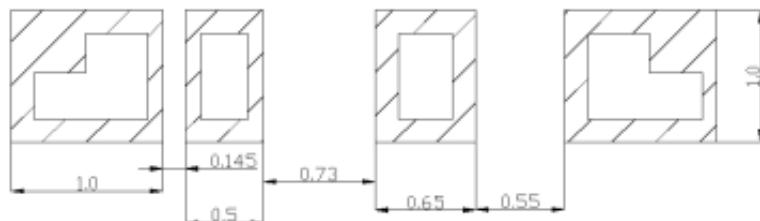
建议焊盘尺寸图:
