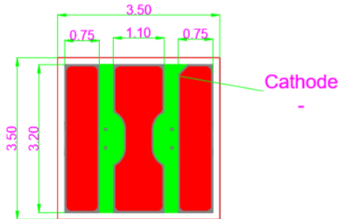
背面图
