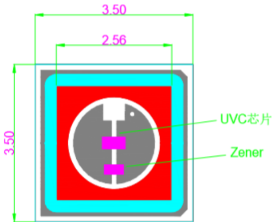
正面图
