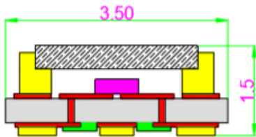
侧面图
